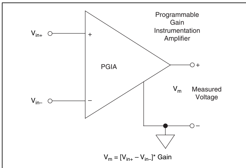
Figure 3-2. DAQPad-MIO-16XE-50 PGIA
