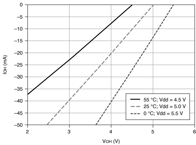
Figure 5. PFI <0..15>/P1/P2: I_{OH} versus V_{OH}
