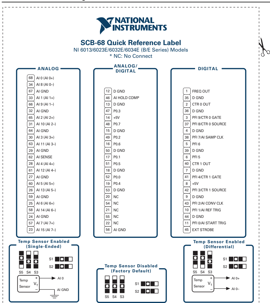
Figure 2. NI 6013/6023E/6032E/6034E
