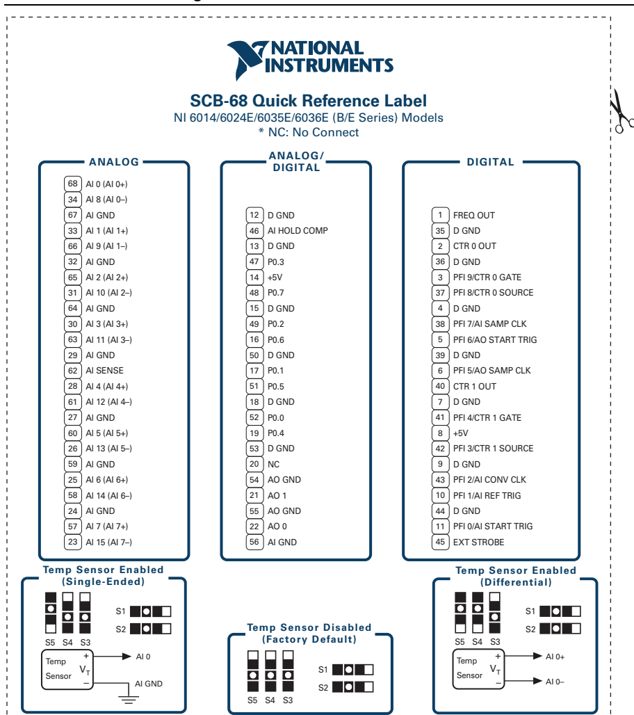
Figure 3. NI 6014/6024E/6035E/6036E
