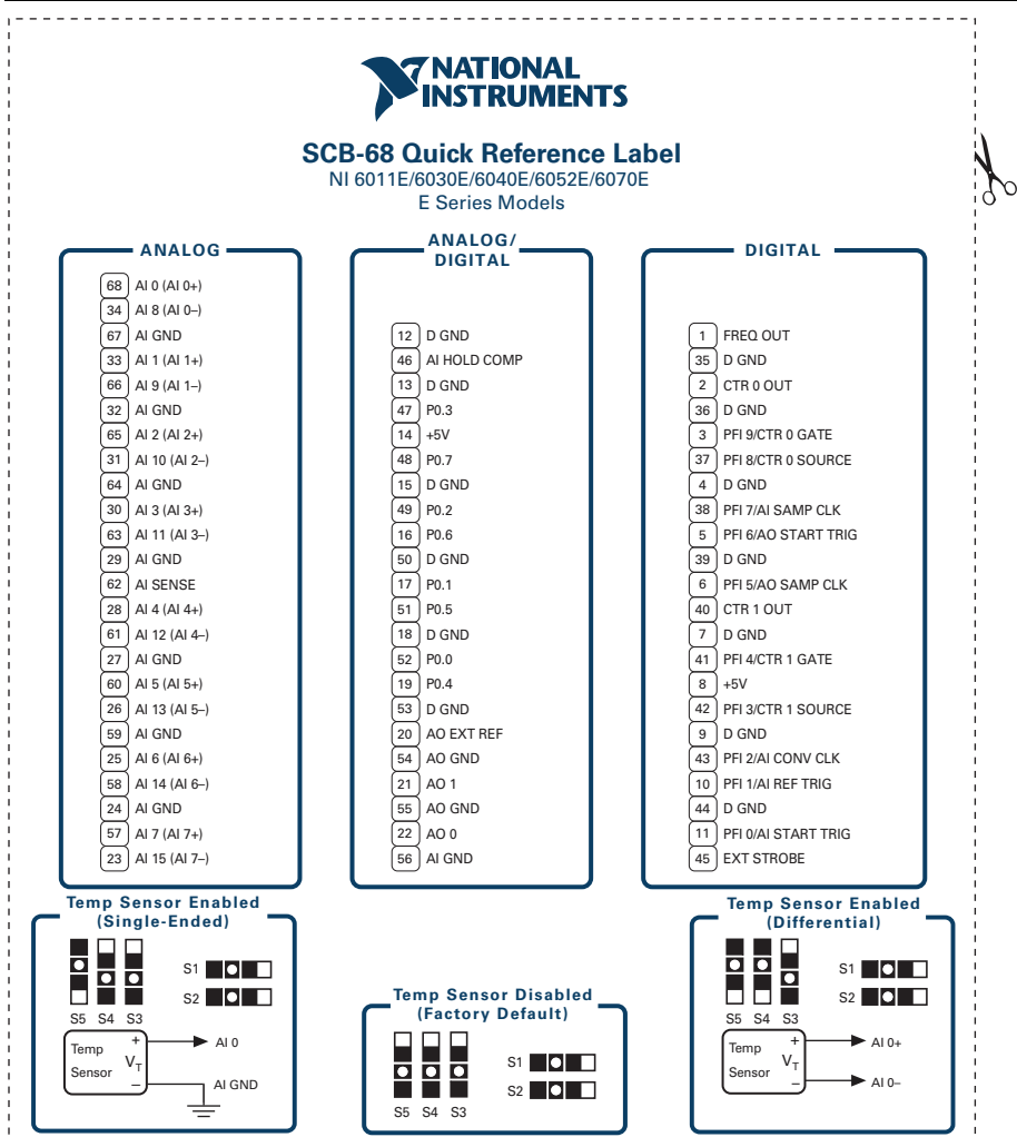
Figure 1. NI 6011E/6030E/6040E/6052E/6070E
