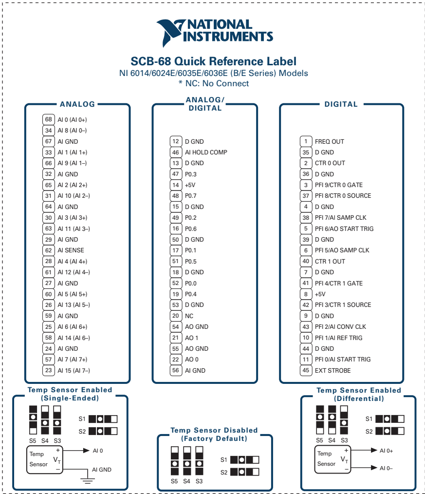
Figure 3. NI 6014/6024E/6035E/6036E
