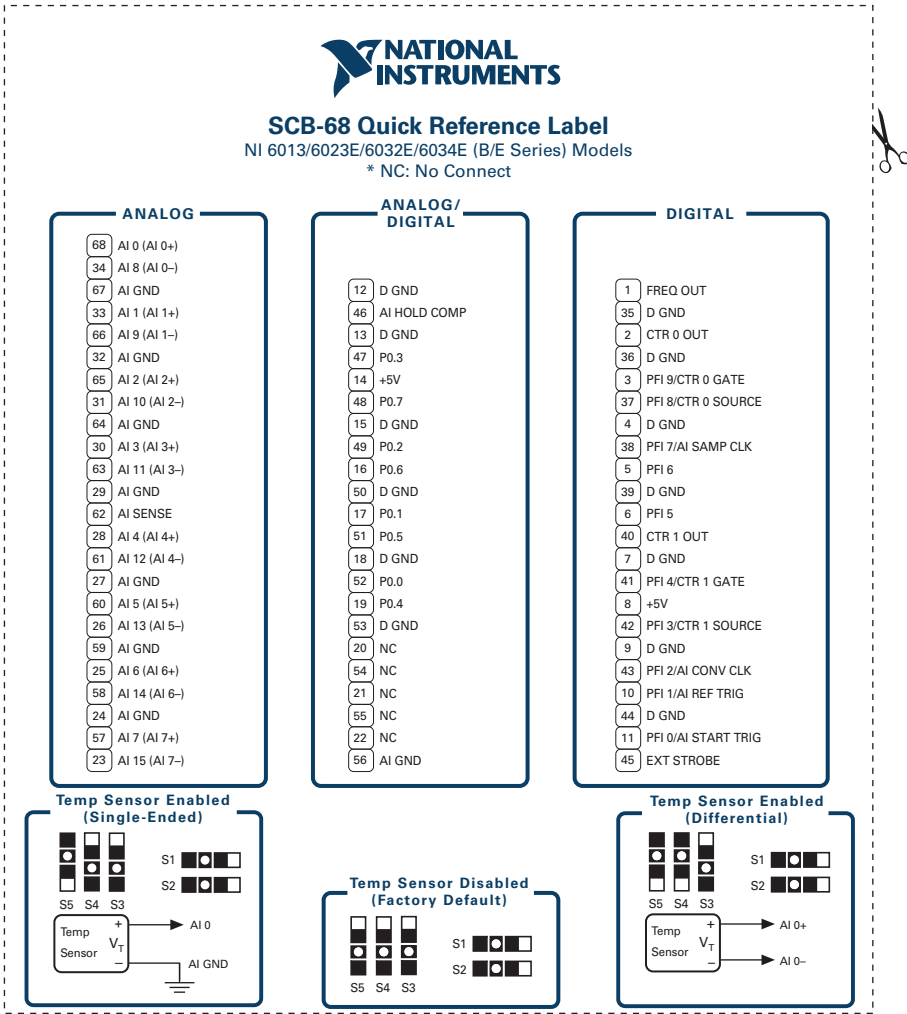
Figure 2. NI 6013/6023E/6032E/6034E
