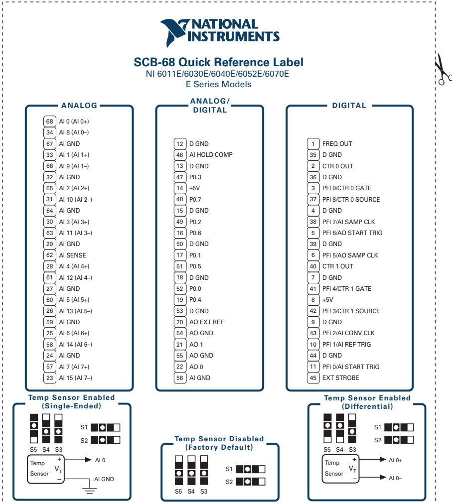
Figure 1. NI 6011E/6030E/6040E/6052E/6070E
