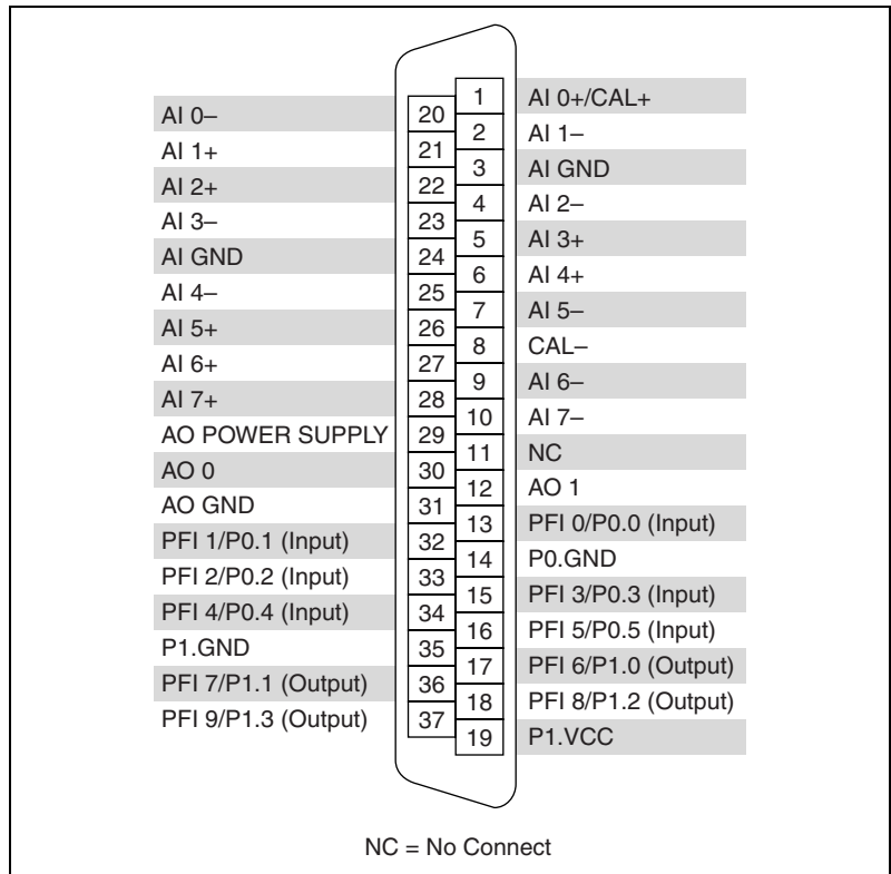
Figure A-2. NI 6239 Pinout
