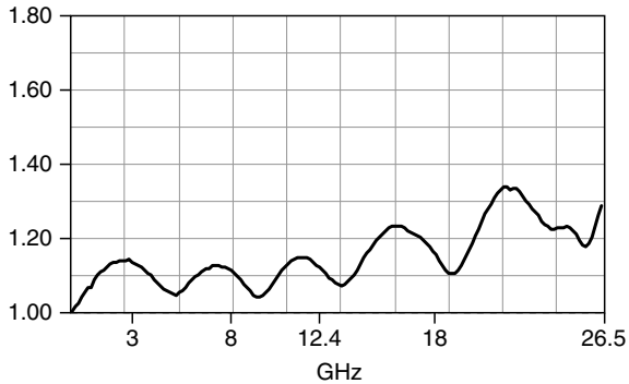
図 2. VSWR (標準)
