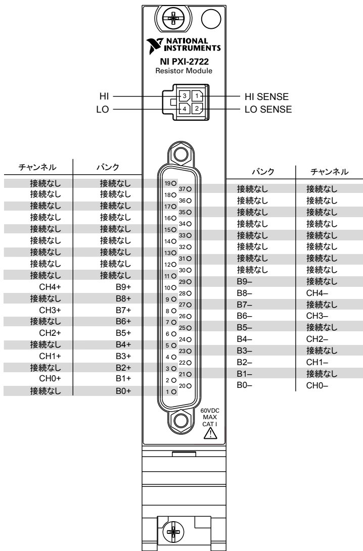
図 5. NI 2722 コネクタのピン配列
