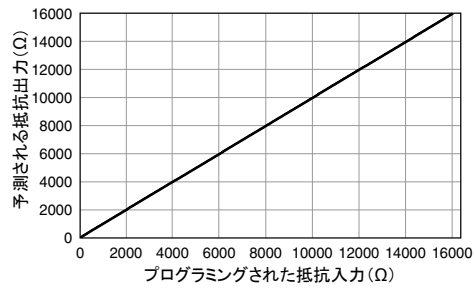
図 3. 0 Ω~16,000 Ω での予想される抵抗
