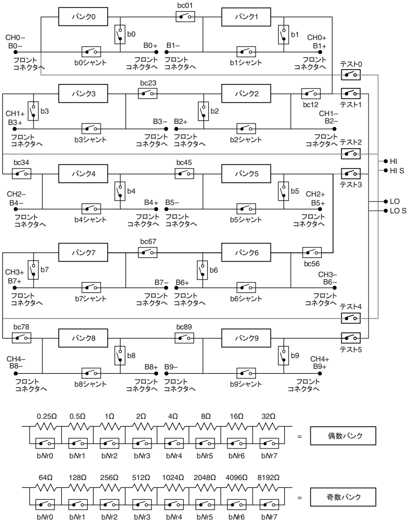
図 6. NI 2722 電源投入時の状態
