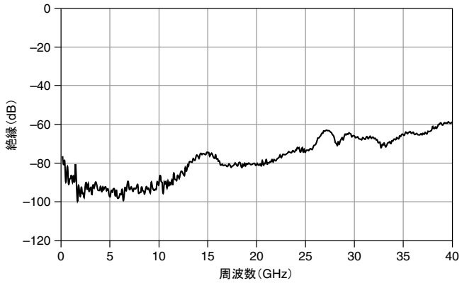
図 2. 標準絶縁
