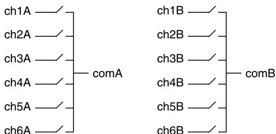
図 4. NI 2796 電源投入時の状態
