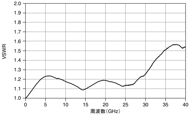
図 3. 標準 VSWR
