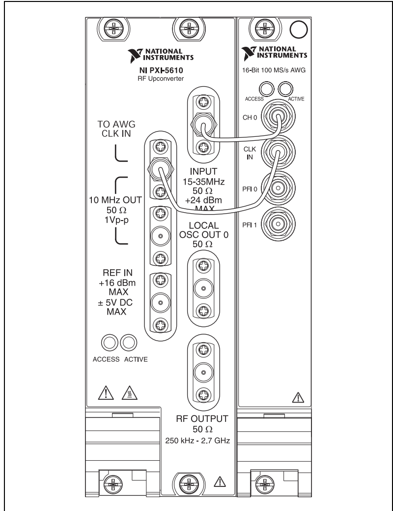
図 7 NI PXIe-5672 フロントパネル
