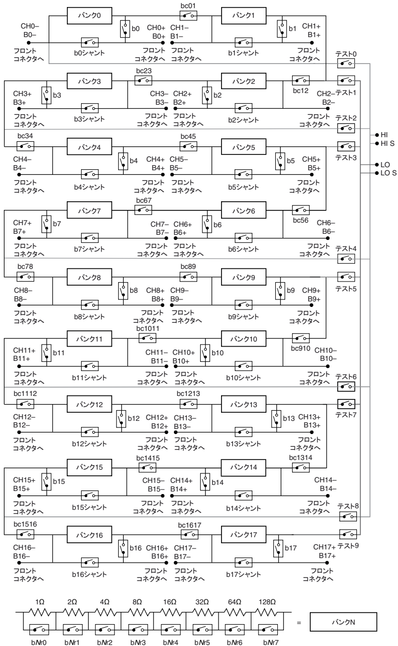
図 4. NI 2725 電源投入時の状態
