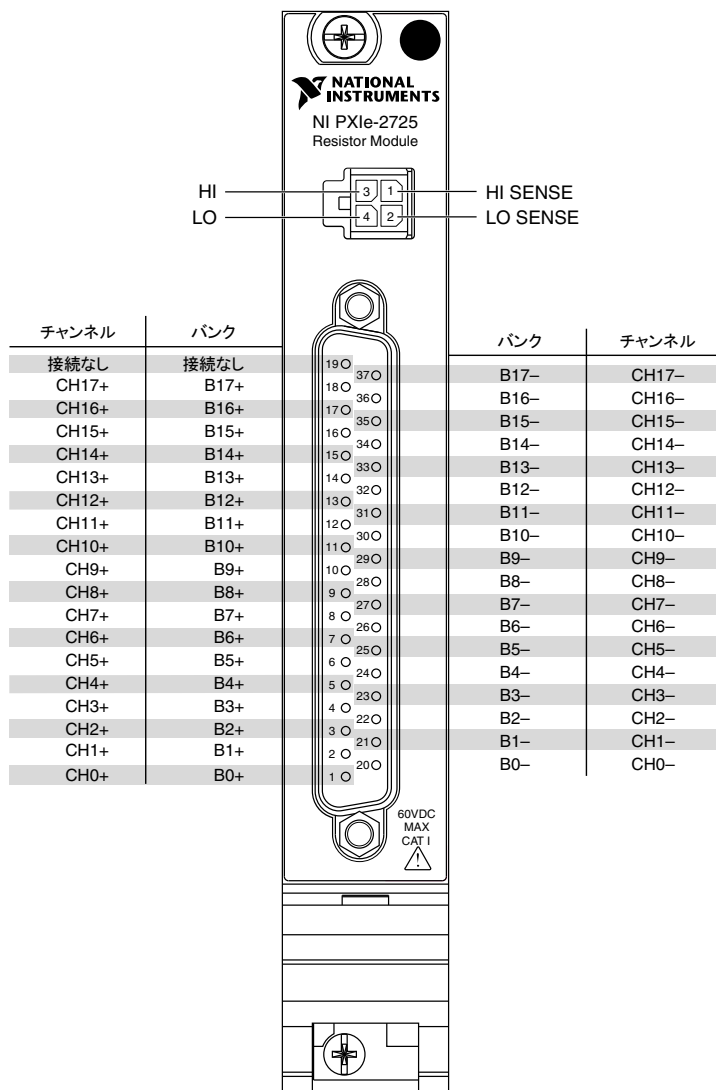
図 3. NI 2725 コネクタのピン配列
