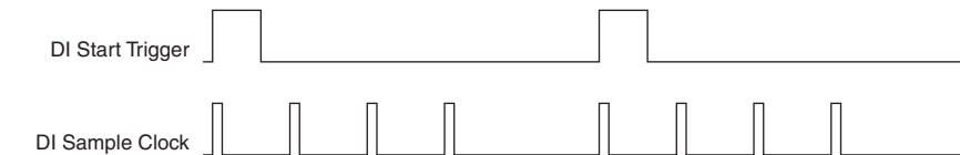
Figure 5-4. Retriggerable DI
