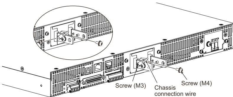
Figure 6. RMX-4122/4123/4126/4127
