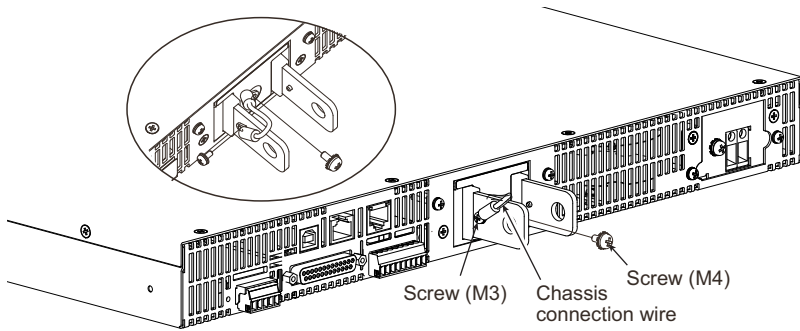
Figure 6. RMX-4122/4123/4126/4127
