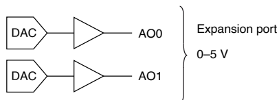
Figure 29. AO Circuitry
