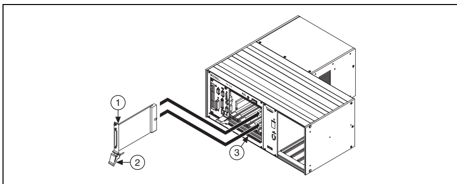
1 Module DAQ PXI 2 Dispositif d'insertion/éjection 3 Rail d'insertion/éjection
