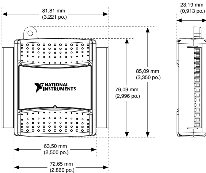
Figure 1. Dimensions de l'USB-6008
