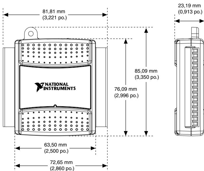
Figure 1. Dimensions de l'USB-6009
