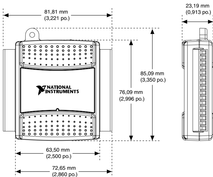
Figure 1. Dimensions de l'USB-6009
