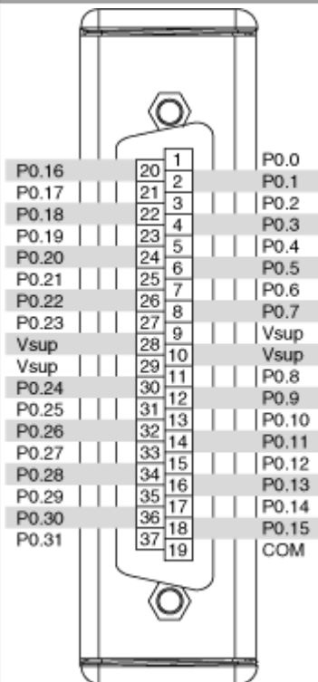
NI 9476 DSUB
