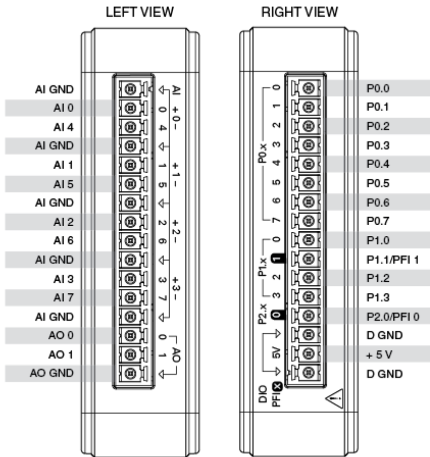
USB-6003
