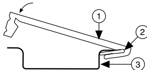
Figure 31. DIN Rail Clip Parts Locator
